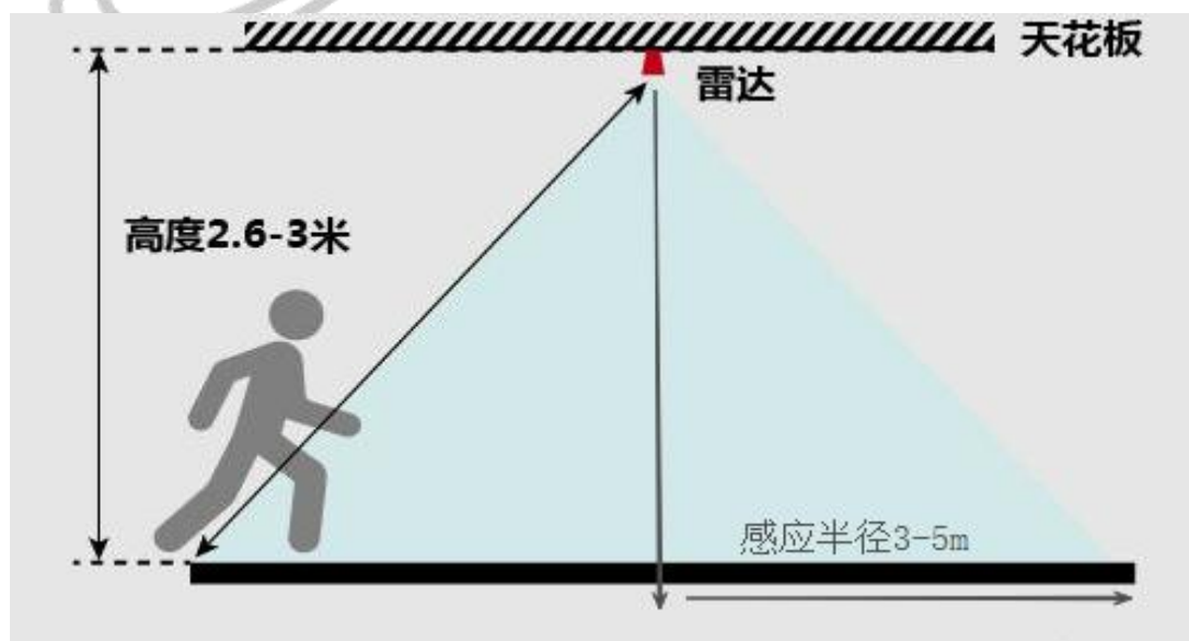
挂高探测图
